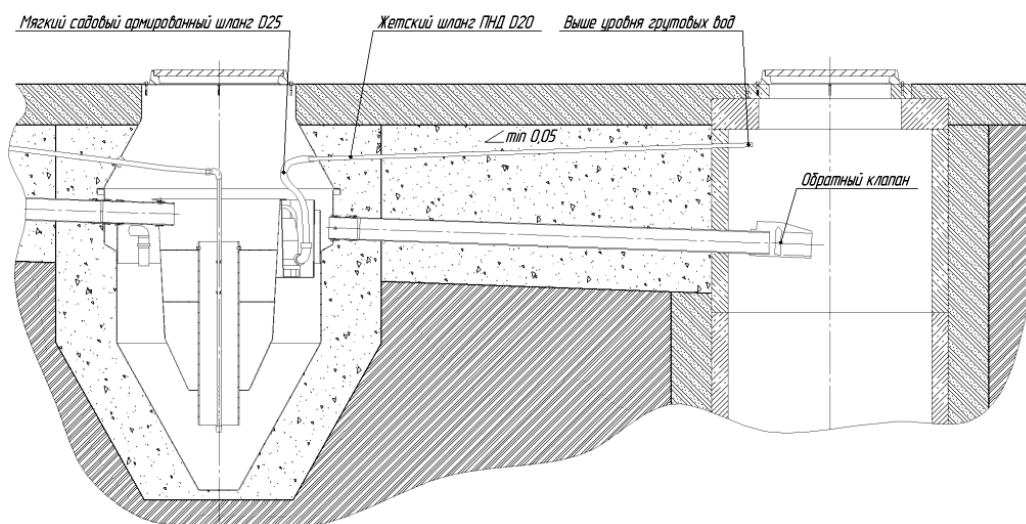
Рисунок 9 - Монтаж Станции с Комплектом ПР
