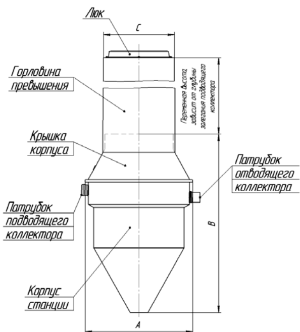
Рисунок 2 - Габаритные размеры и основные части Станции
