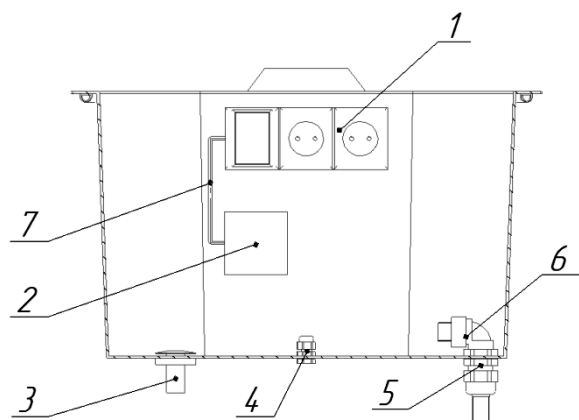
Рисунок 11 - Монтаж Станции с Коробом компрессора
