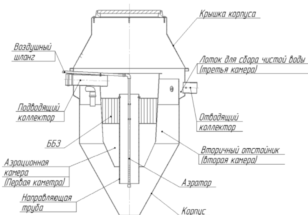
Рисунок 1 – Элементы Станции
