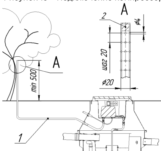
Рисунок 14 - Установка воздуховода
